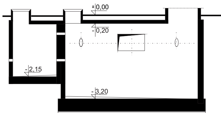
PRZEKRÓJ
