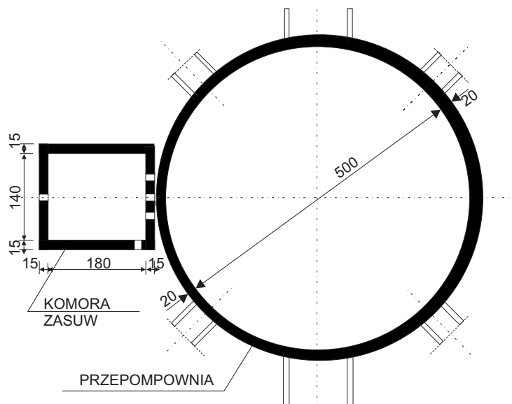
RZUT
